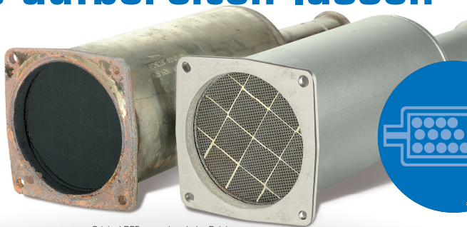
Original DPF vor und nach der Reinigung
